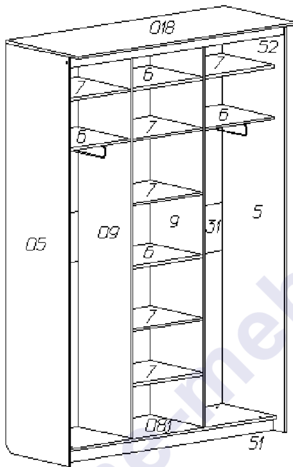
Комплектовочная ведомость деталей
